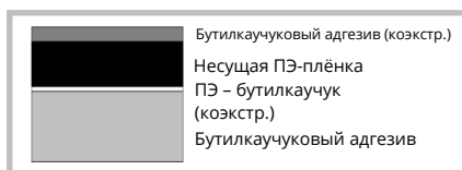
DENSOLEN®-AS40 Plus
